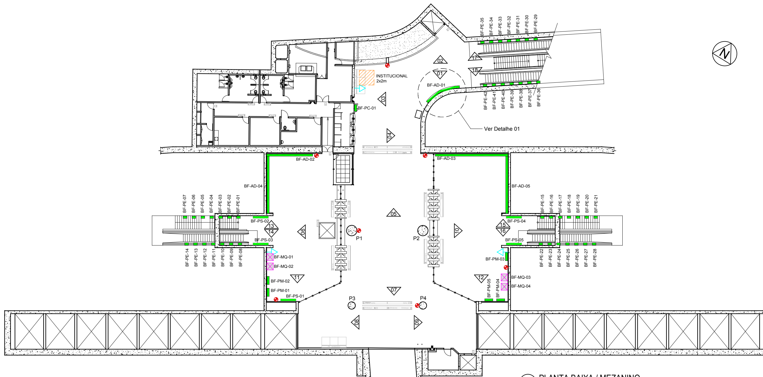
01 PLANTA BAIXA / MEZANINO ESC.: 1/30
