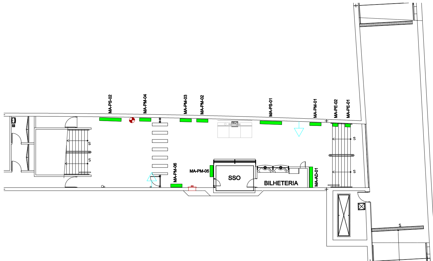
01 PLANTA BAIXA / MEZANINO ESC.: 1/15
