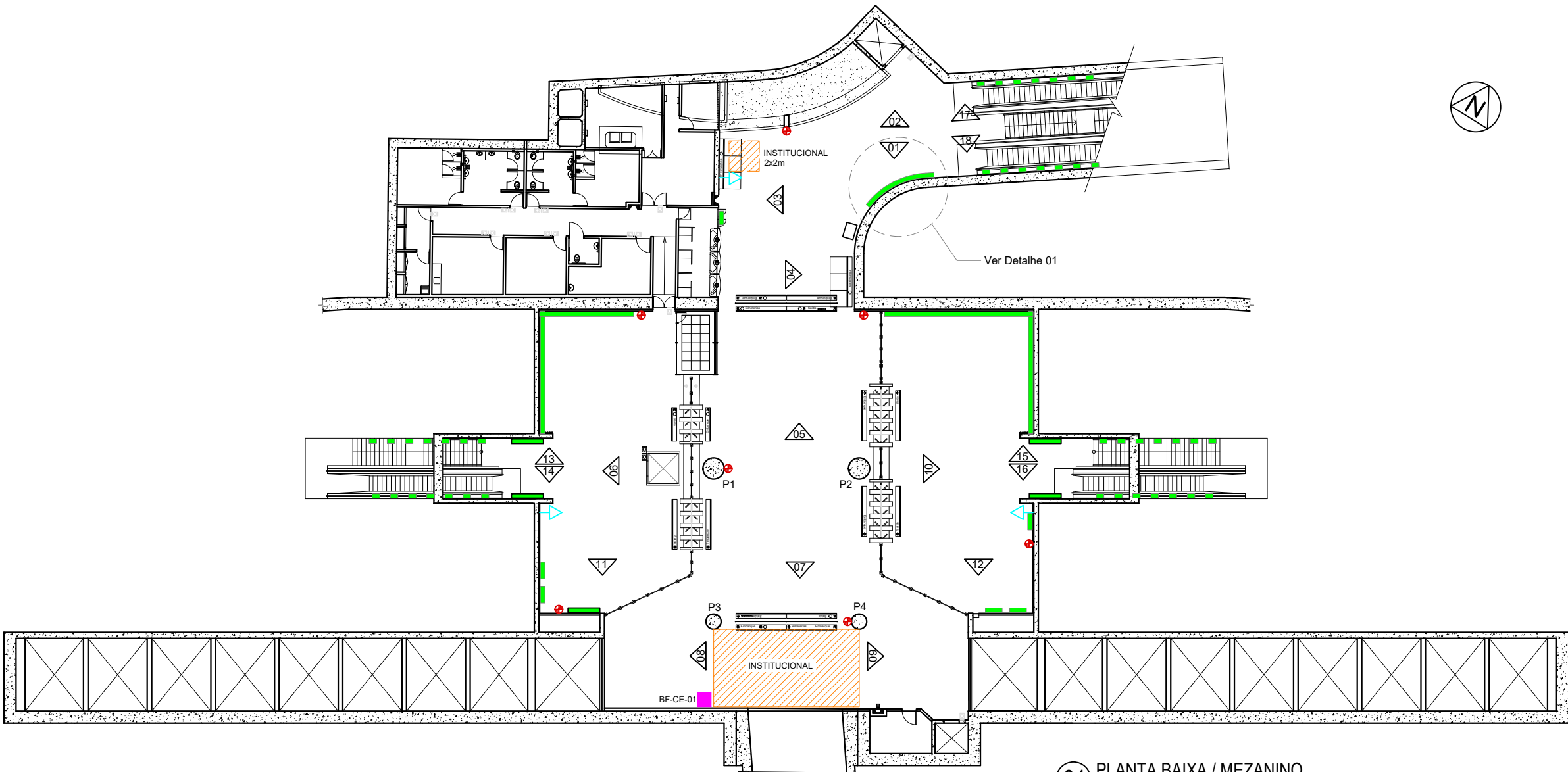
01 PLANTA BAIXA / MEZANINO ESC.: 1/30
