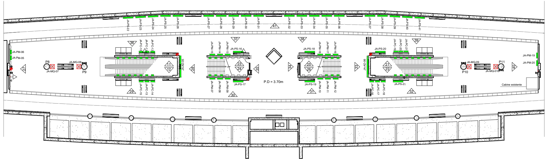
01 PLANTA BAIXA / PLATAFORMA ESC.: 1/30
