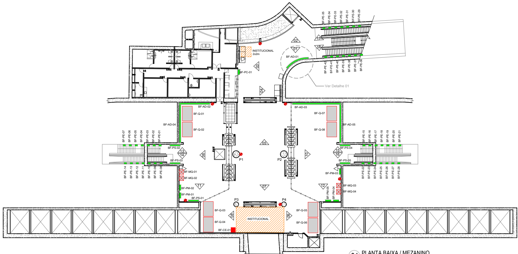
01 PLANTA BAIXA / MEZANINO ESC.: 1/30
