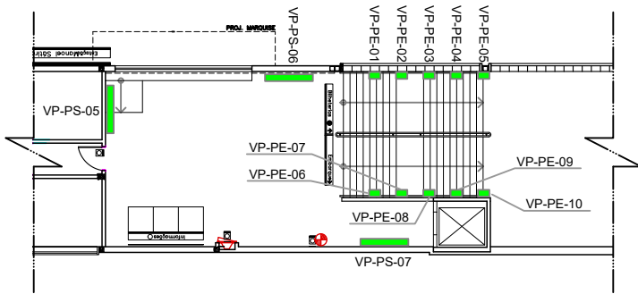
01 PLANTA BAIXA / TÉRREO ESC.: 1/20
