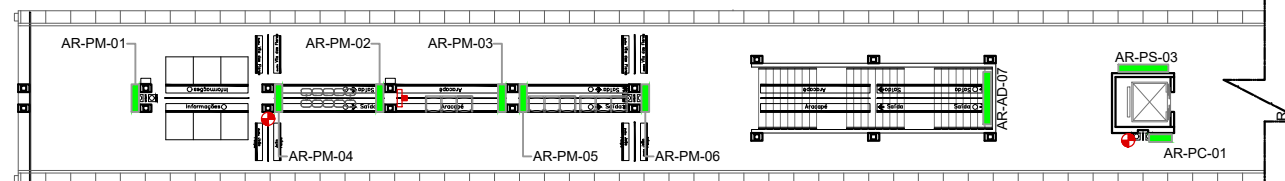
01 PLANTA BAIXA / PLATAFORMA ESC.: 1/20
