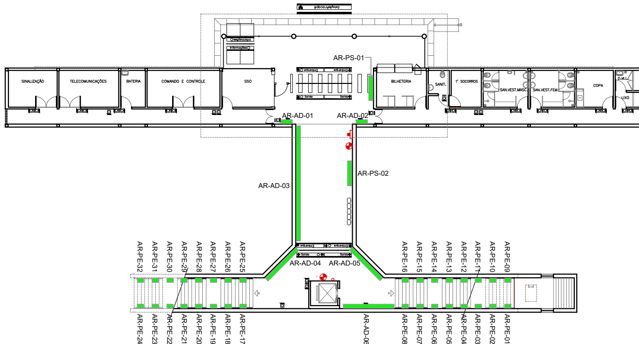
01 PLANTA BAIXA / TÉRREO ESC.: 1/20
