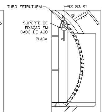
04 CORTE 02 ESC.: 1/5
