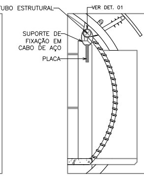
05 CORTE 03 ESC.: 1/5
