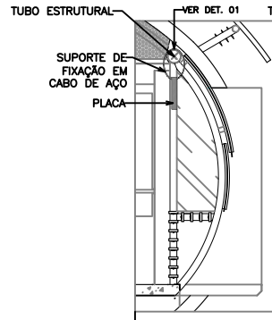
03 CORTE 01 ESC.: 1/5
