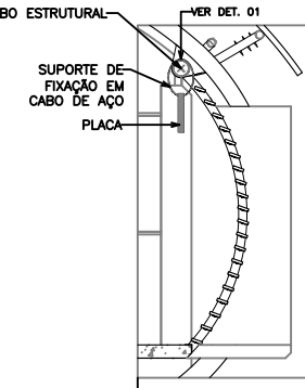
04 CORTE 02 ESC.: 1/5
