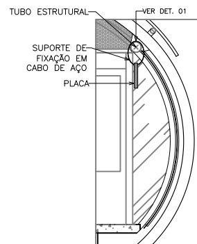
03 CORTE 01 ESC.: 1/5
