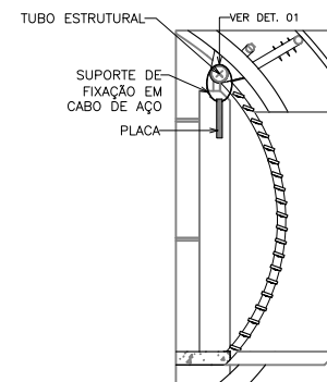
04 CORTE 02 ESC.: 1/5
